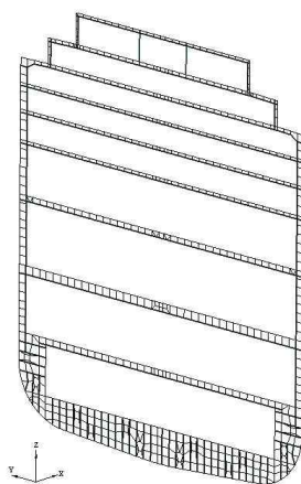
그림 28 특설늑골의 예
