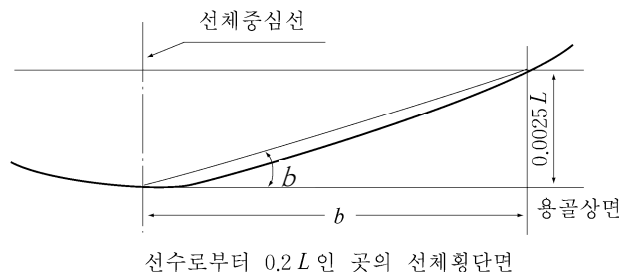
그림 3.7.2 b 의 측정방법
