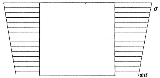
그림 3.2 좌굴응력 보정계수
