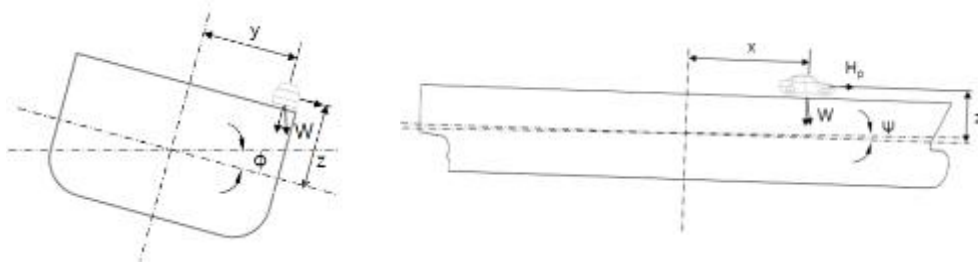
그림 1 선체운동
