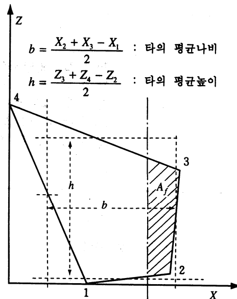
그림 4.1.2 타의 좌표계
