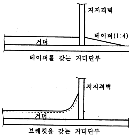
그림 3.5.11 거더의 단부
