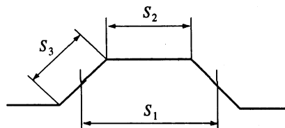
그림 3.3.1 파형격벽
