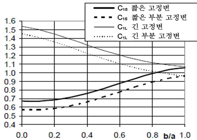
그림 3.5.5 계수 C_1
