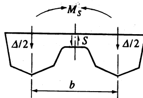
그림 3.2.13 횡방향 수직 굽힘모멘트 및 전단력
