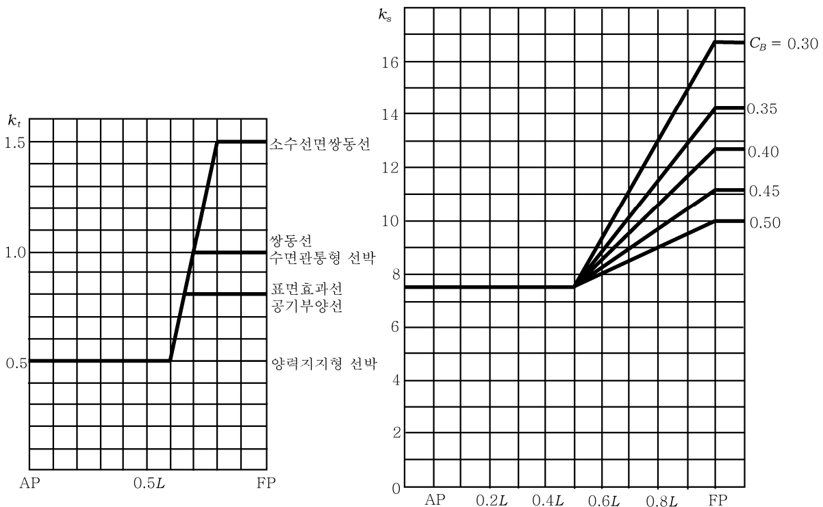
그림 3.2.8 쌍둥선연결부 슬래밍 분포계수 k_t
