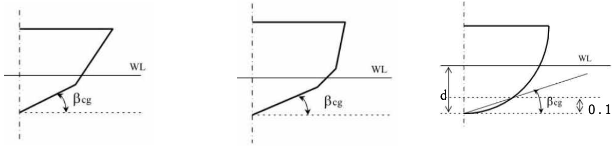
그림 3.2.4 선저각도, \beta_{cg}
