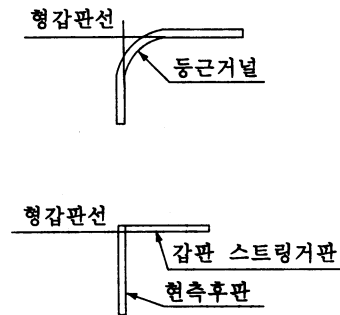
그림 3.3.3 형기준선
