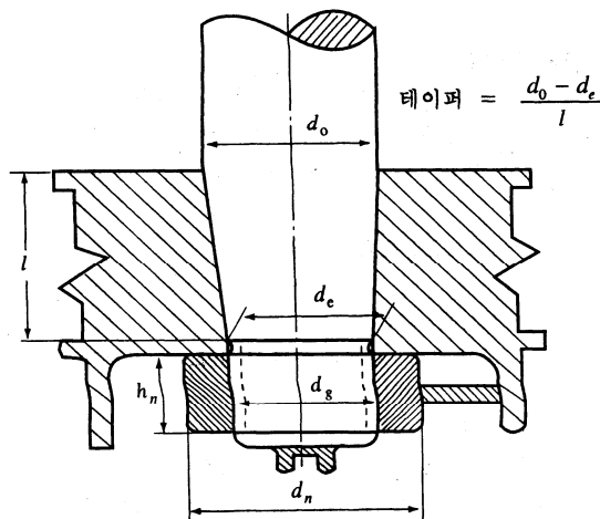
그림 4.1.3 유압장치가 없는 콘 커플링
