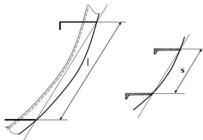
그림 1.2 곡부재에 대한 늪골 스패(왼쪽) 및 늪골 간격(오른쪽)의 정의
