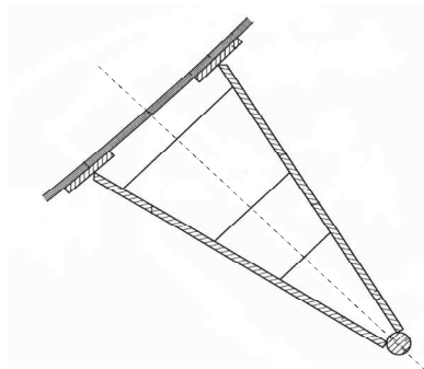
그림 1.6 전형적인 빙지킬의 설계 예
