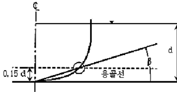
그림 3.2.4 등근 단면의 선저각도
