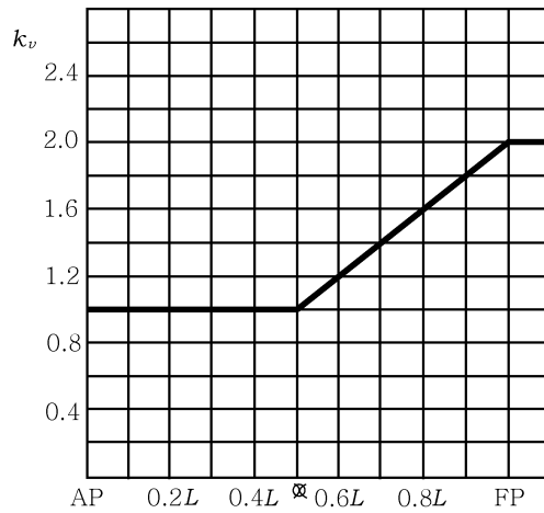
그림 3.2.1 수직설계가속도의 길이방향 분포계수 k_v
