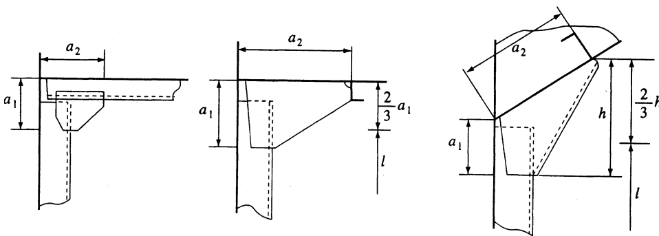
그림 3.3.4 브래킷의 치수
