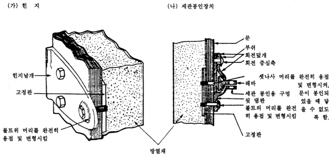
그림 1 방열컨테이너 문의 부착 예
