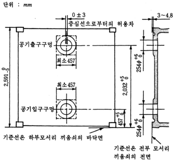
그림 2.24 1CC 방열 컨테이너 단부벽의 공기구멍
