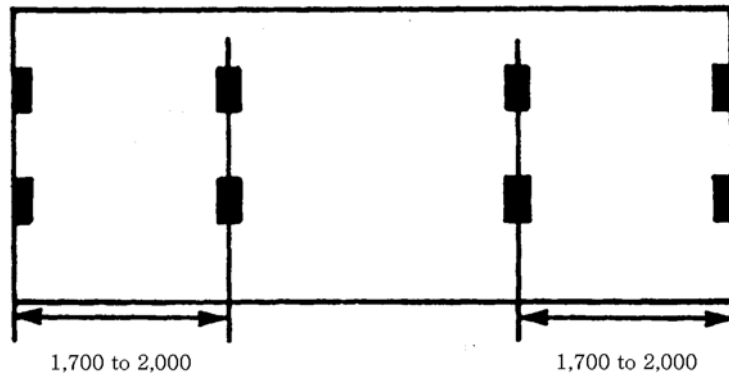
그림 2.12 1CC, 1C 또는 1X 컨테이너의 바닥구조 하중전달면 (단 : mm)
