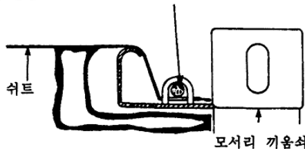
(나) 단면도 슈트 고정용 패스닝(로프)
