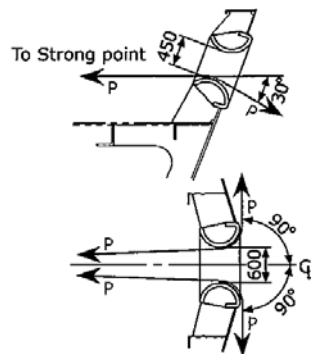
그림 3.7.1 하중시험 방향
