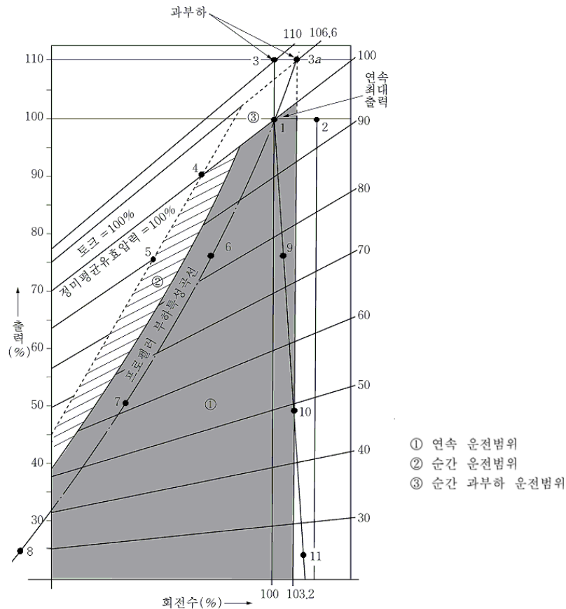
그림 3.8.1 부하설정점
