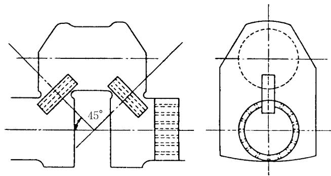
그림 2.5.3 굽힘피로시험편 채취위치
