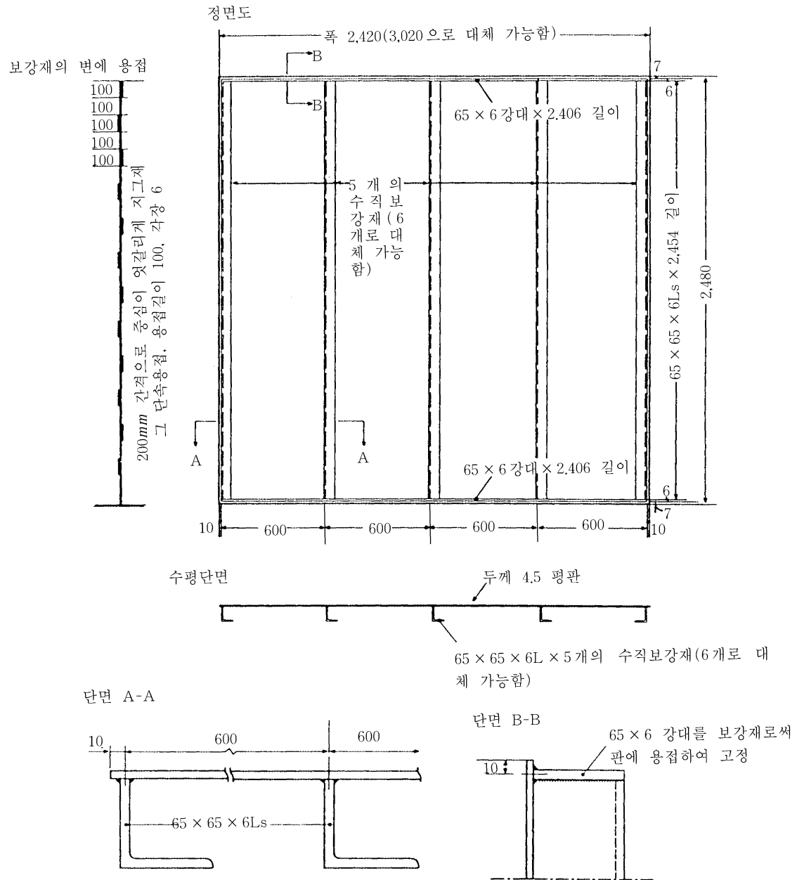
그림 3.26.2 A급 격벽 및 B급 내장재의 주요구조부재의 치수
