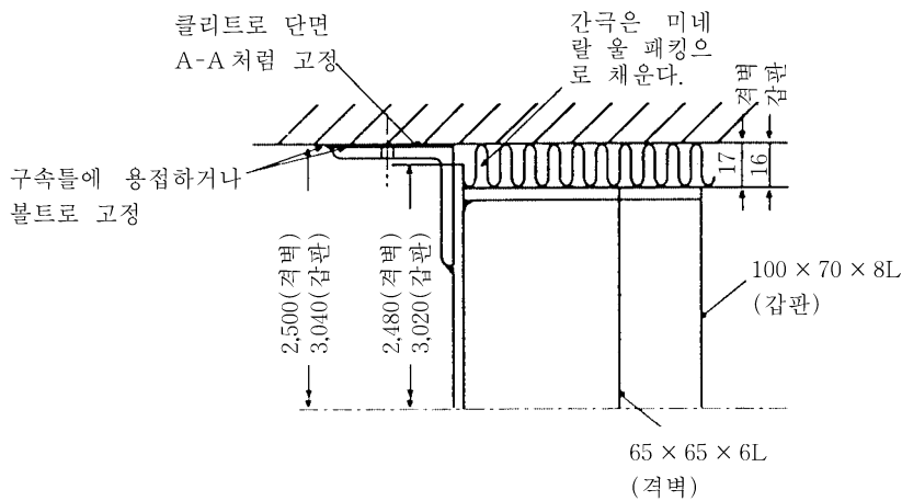
그림 3.26.3 구속틀과 주요구조부재의 결
