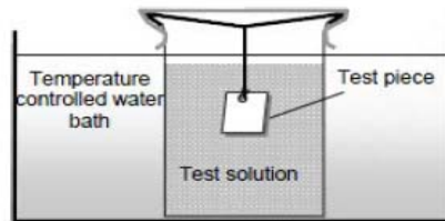
그림 3.32.6 내저판용 모의 부식시험장치
