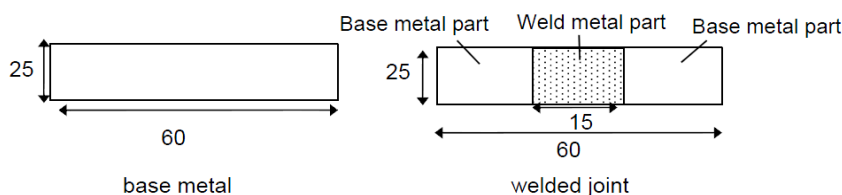
그림 3.32.1 시험편의 치수
