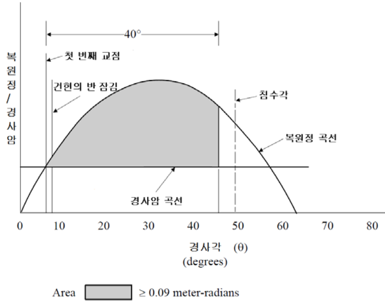
그림 8.2 복원정 및 경사면 곡선
