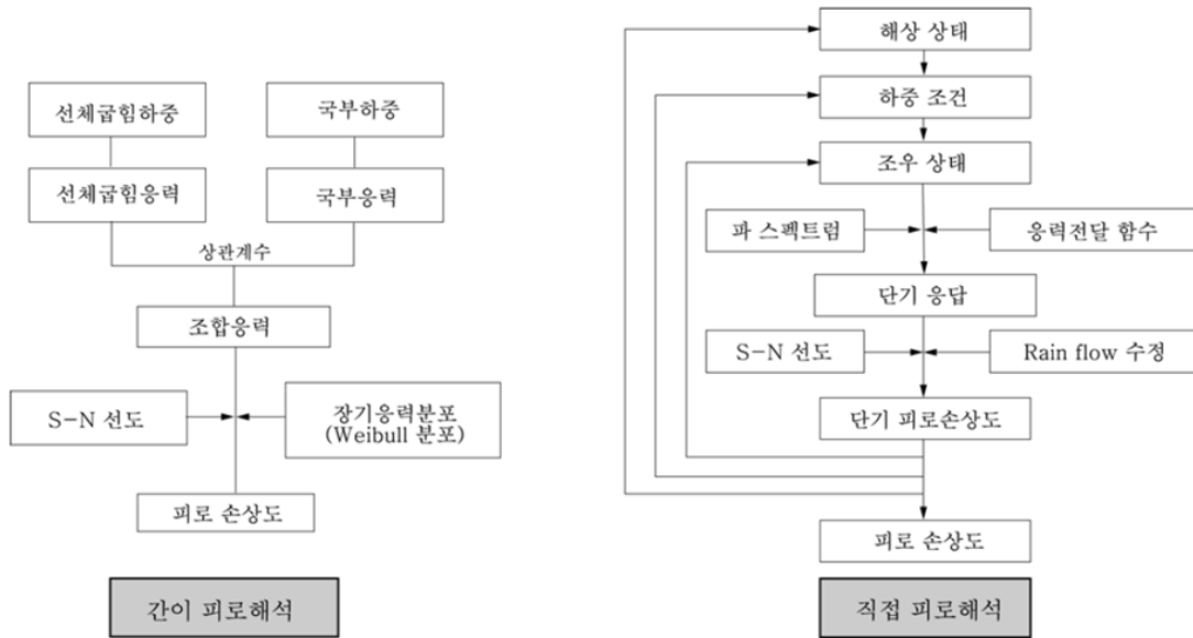
그림 5.2 피로해석 방법
