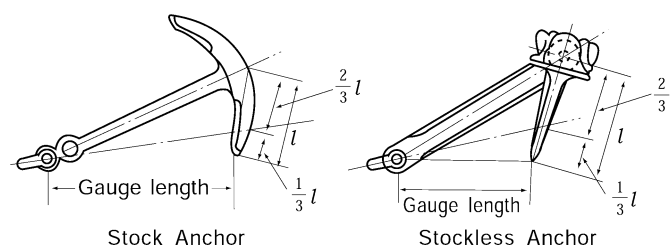
Fig 4.8.1 Anchors
